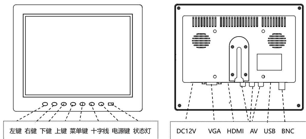
显示屏正、反面功能接口说明
