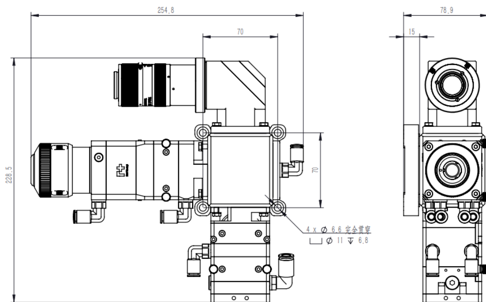
准直 F100/带视觉镜头 90°样式尺寸
