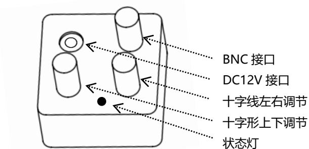
相机功能接口说明
