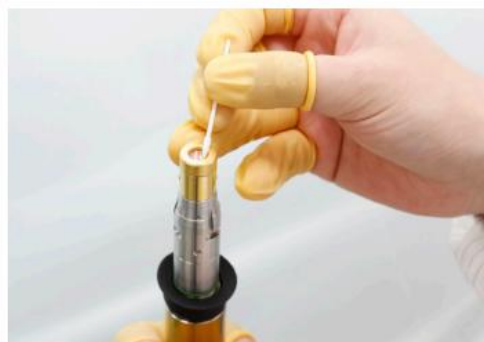
棉签擦拭保护镜片
