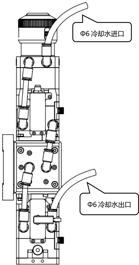
BW06K 激光焊接头冷却水接法
