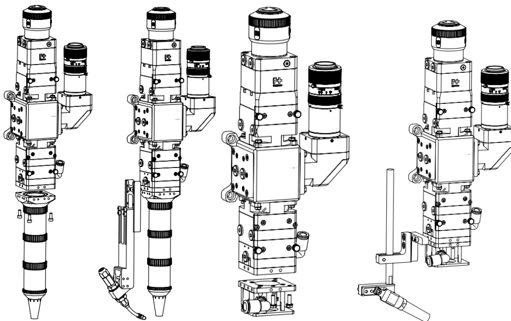
(F300)同轴吹气组件
