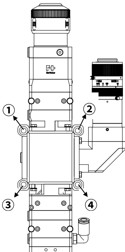
BW06K 正视图
